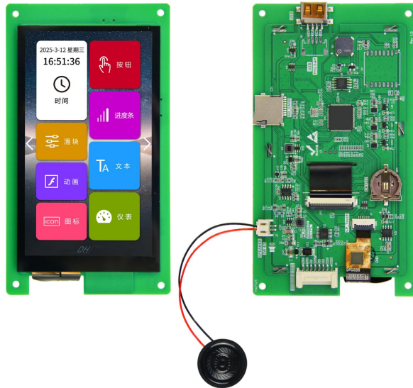
图 1-1 5.0 寸电容触摸参考图
