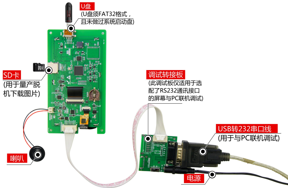
图 1-4 调试工具图
