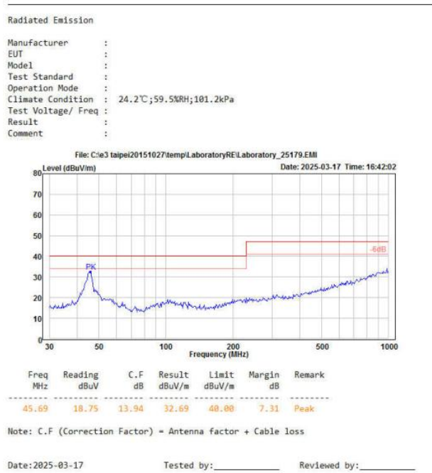
图 5-7 辐射测试垂直方向
